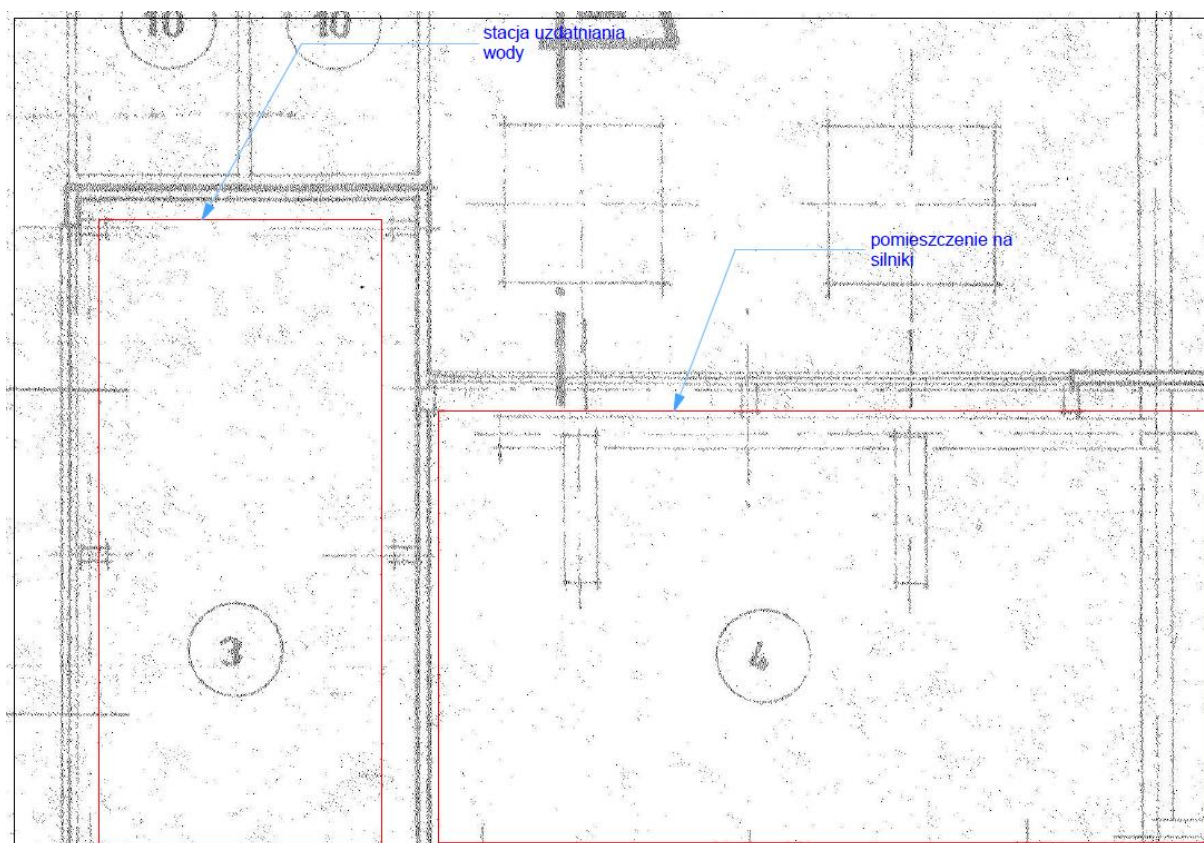
Rysunek 3. Proponowana lokalizacja Instalacji kogeneracyjnej z silnikami gazowymi
