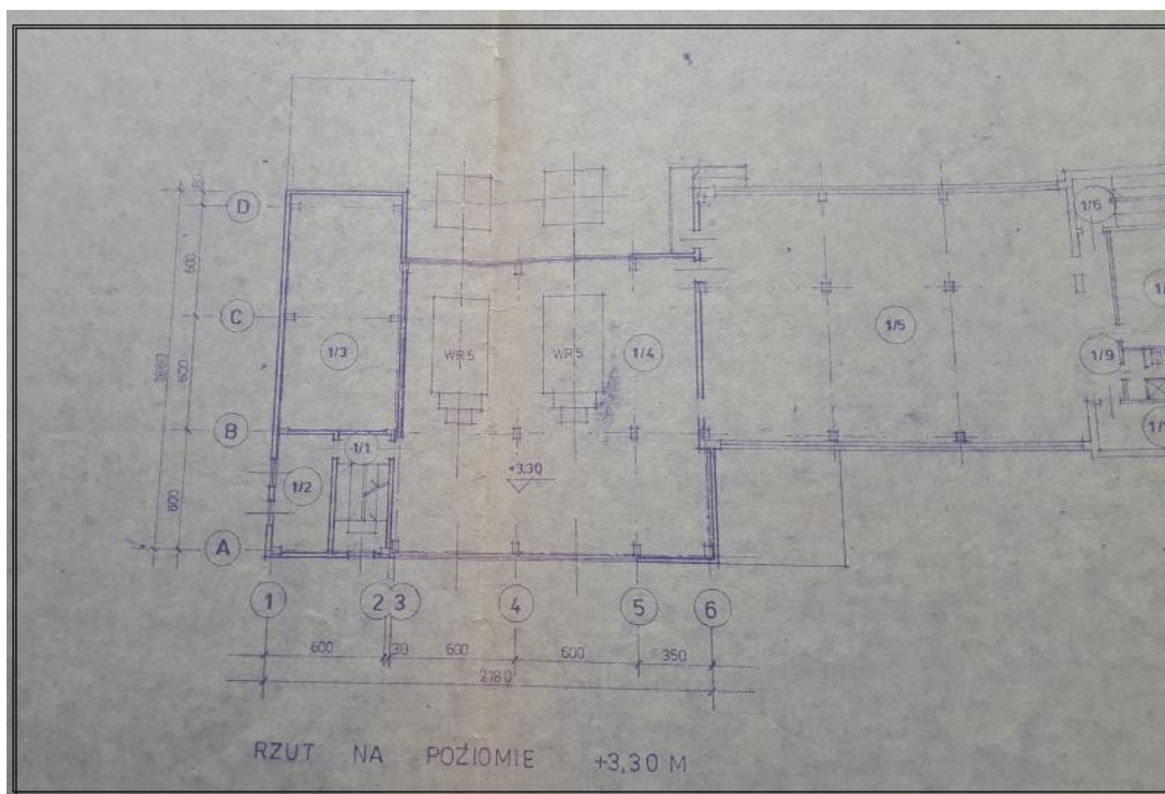
Rysunek 9. Rzut poziom +3,3 m
